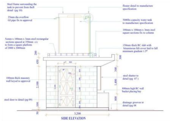
1:1 SIDE ELEVATION 001
